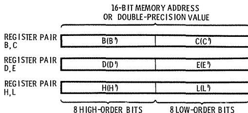
Fig. 2-4. Register pairs.
